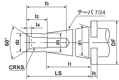
図2 ナショナルテーパ
