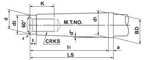
図4 モールステーパ (ねじ付きシャンク)
